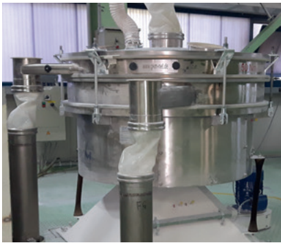
Taumel- /Vibrationssiebe
